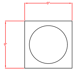
SECTION 01 SCALE: 1 1/2" = 1'-0"
