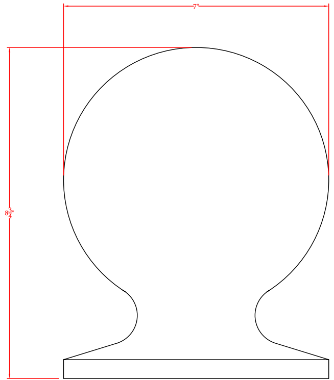
ELEVATION 01 SCALE: 6" = 1'-0"
